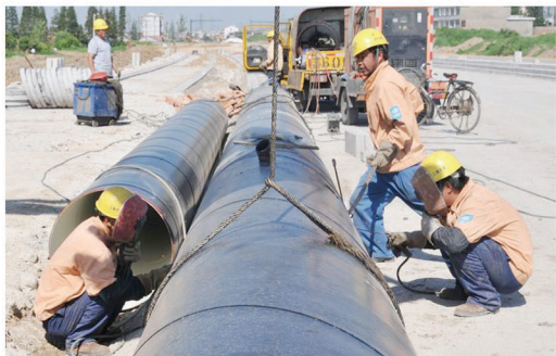
延陵东路DN800管施工现场
