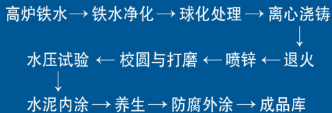
球墨铸铁管生产工艺流程图
